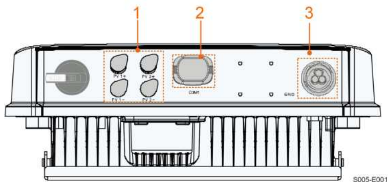
Figura 5-1 Terminais (SG3.0RS-L, por exemplo)
