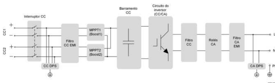
Figura 2-5 Diagrama do circuito (SG6.0RS-L, por exemplo)
