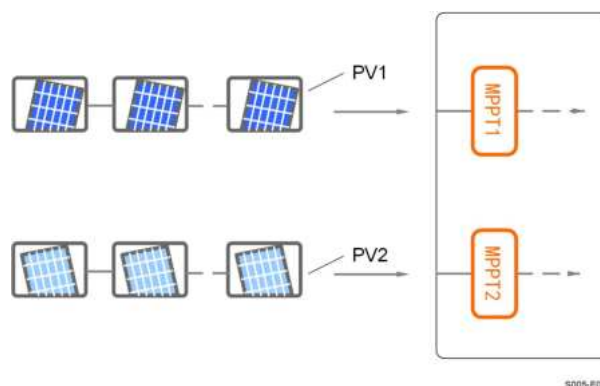
Figura 5-2 Configuração de entrada FV (SG6.0RS-L, por exemplo)
